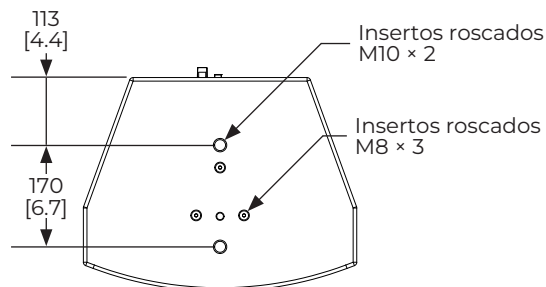
Vista inferior
