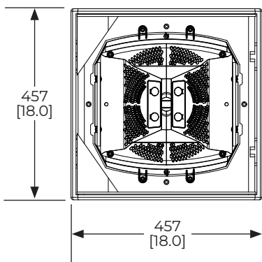
Vista frontal (sin rejilla)
