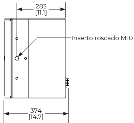
Vista derecha 7
